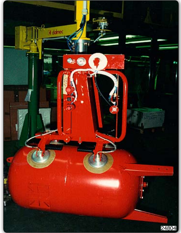
Manipulator with suction cups tooling (Venturi) for gripping and inclination of tanks. 装备真空吸盘 (文丘里) 的机械手臂, 用于抓取和倾斜油箱。
