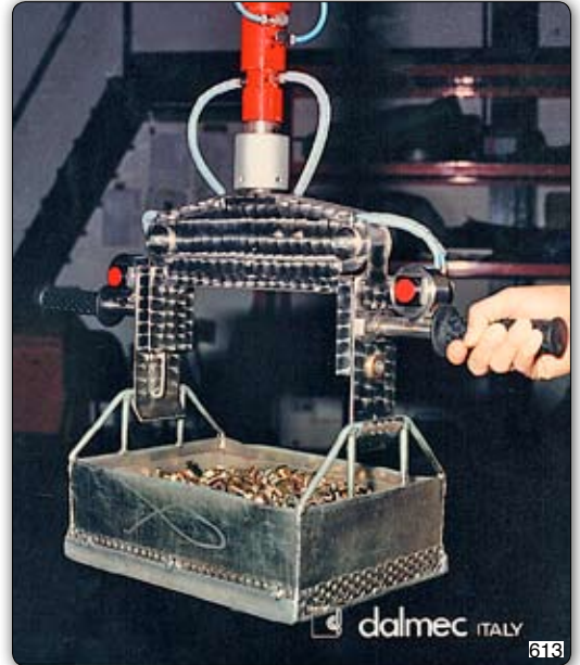
Ruční manipulátor se speciálními háky z nerezavějící oceli pro manipulaci s přepravkami.
