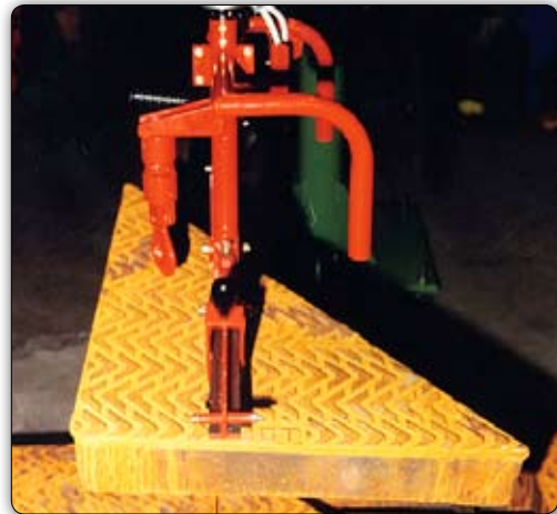
Ruční manipulátor „Partner“ typ PMC, sloupový přístroj, s úchopním zařízením k manipulaci s litinovými poklopy.
