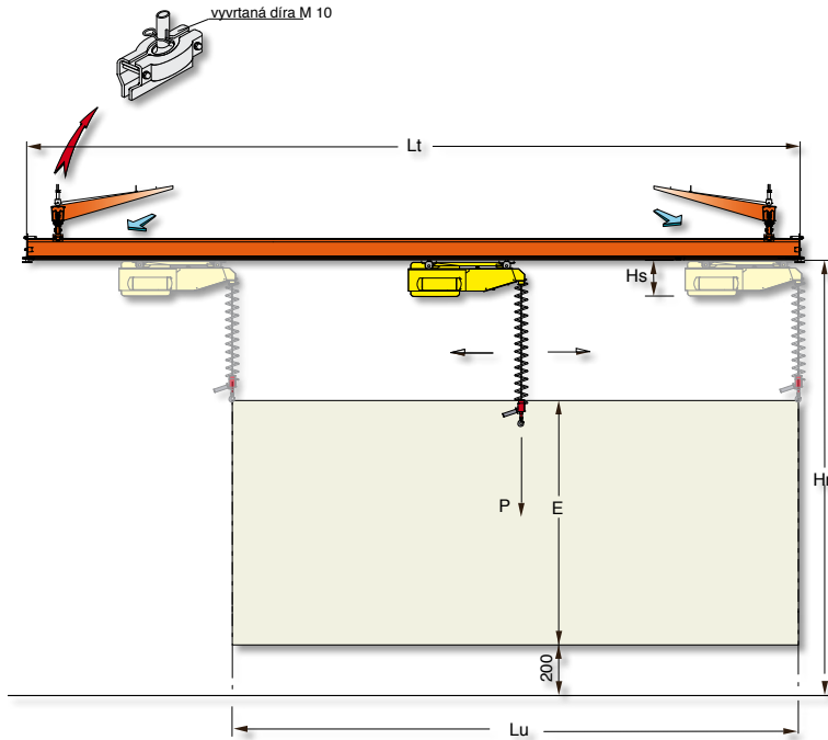
MINIPARTNER stropní přístroj pojízdní „MPS“
