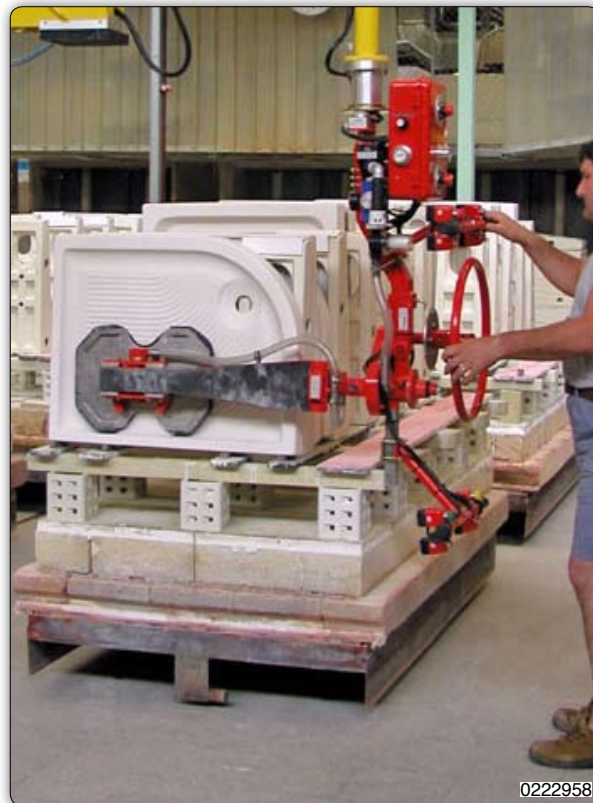
Ruční manipulátor „Partner“ typ PMF, stropní přístroj, s přísavním zařízením (Venturi) k uchopení a ručnímu otáčení sprchových van. 0222958
