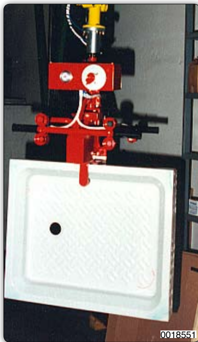
Ruční manipulátor s pneumatickým drapákem k uchopení a otáčení sprchových van. 0018551
