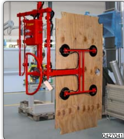
Ruční manipulátor s přísavným zařízením k uchopení a ručnímu otáčení dřevěných panelů.
