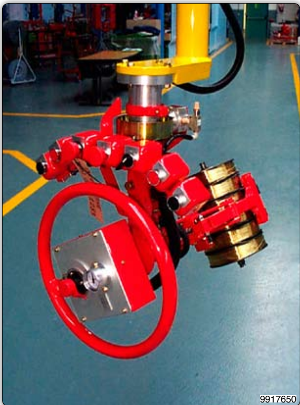
Ruční manipulátor se speciálním drapákem pro uchopení mnohonásobné cívký. Ruční otáčení o 90°.
