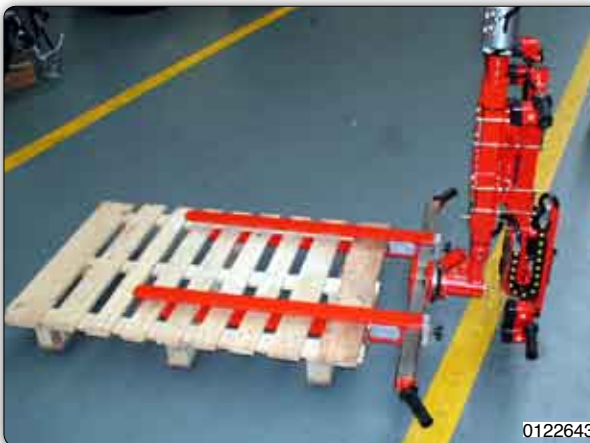
Gabelvorrichtung mit teleskopierbaren Bedienelementen zur Handhabung von Paletten.
