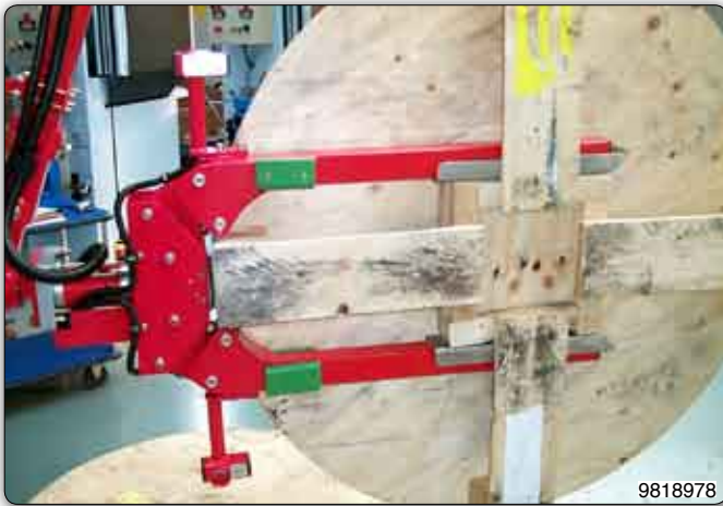
Handhabungs-Manipulator mit Greifvorrichtung und manueller Drehung von speziellen Paletten.
