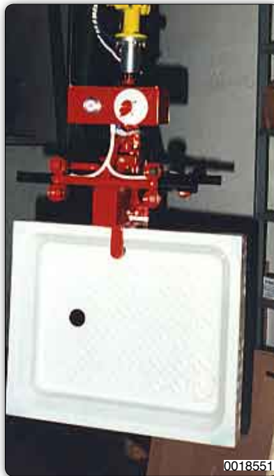
Handhabungs-Manipulator mit pneumatischer Greifvorrichtung zur Handhabung der Duschplatten.
