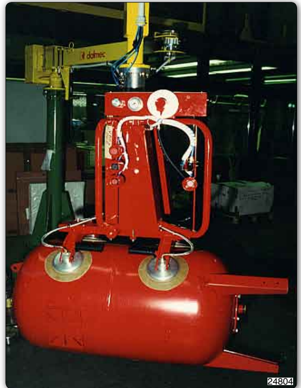
Manipulador con implemento a ventosa (Venturi) para la toma y la inclinación de depósitos.
