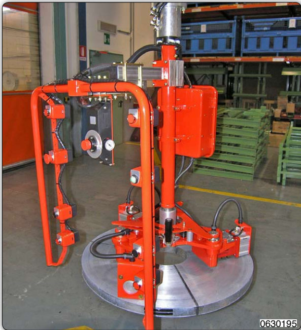
Manipolatore con attrezzo a magneti permanenti multipolari ad azionamento pneumatico, con interasse regolabile manualmente, per la presa ed il sollevamento di rotoli bandella acciaio.
