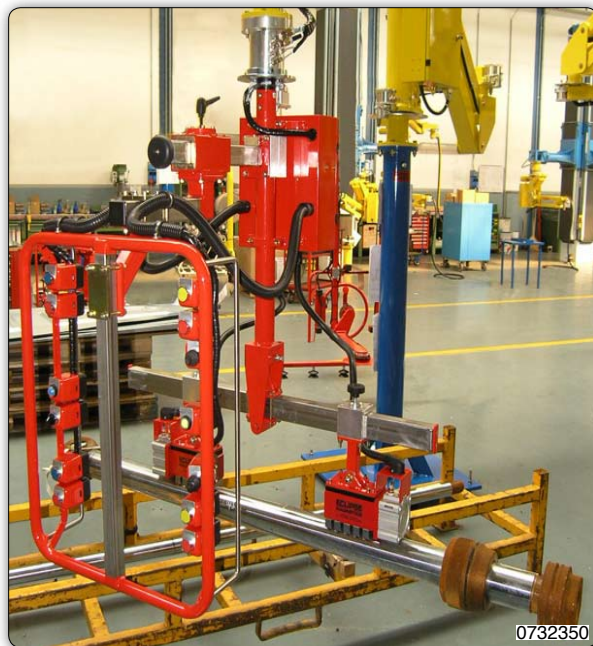
Manipolatore con attrezzo a magneti permanenti multipolari ad azionamento pneumatico, per la presa ed il sollevamento di alberi in acciaio.
