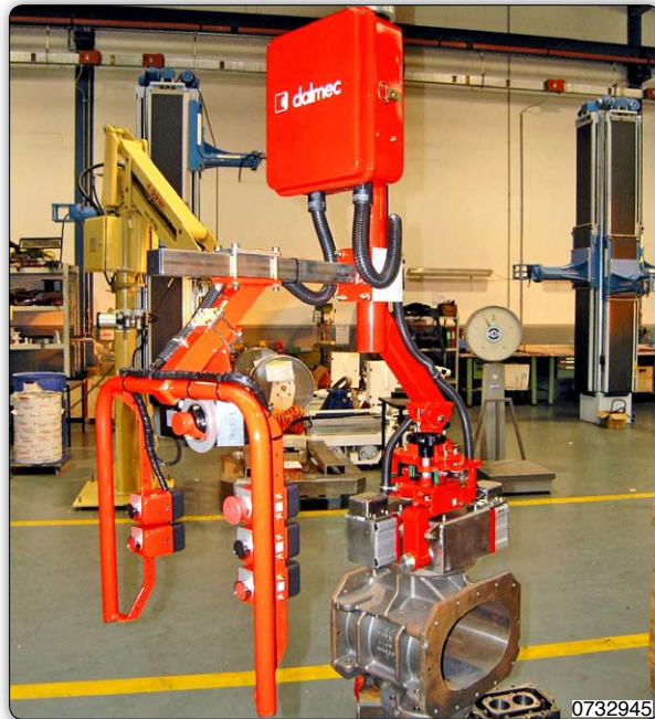
Manipolatore con attrezzo a magneti permanenti multipolari ad azionamento pneumatico, per la presa ed il sollevamento di manufatti in acciaio.
