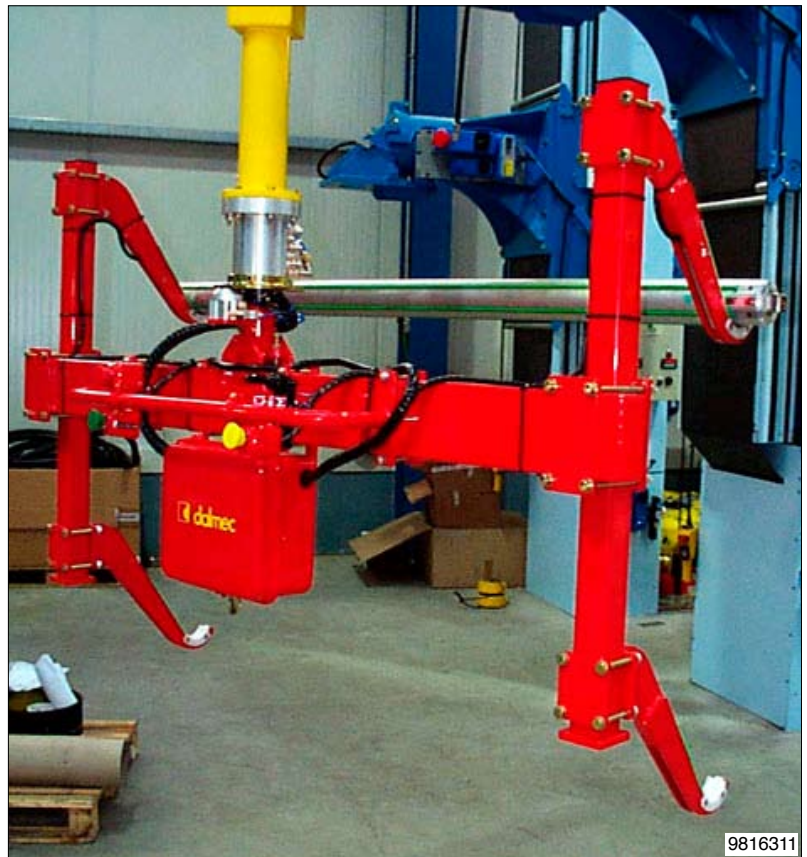
Manipolatore con attrezzo a doppia forca per movimentazione di alberi portabobine.
