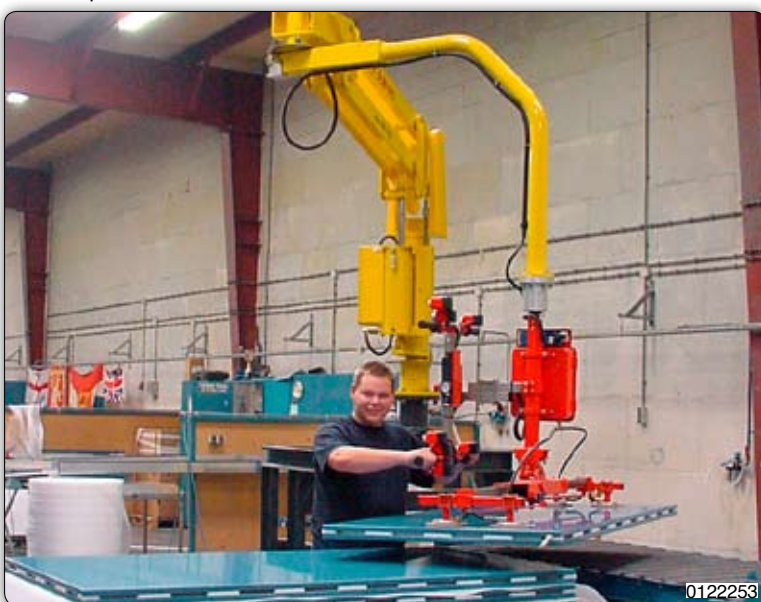
Манипулятор Partner типа PMC в исполнении на стойке, оборудованный приспособлением с регулируемыми присосами для перемещения панелей.
