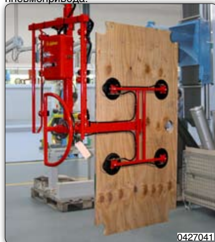
Приспособление с присосами для перемещения деревянных панелей с ручным поворотом.
