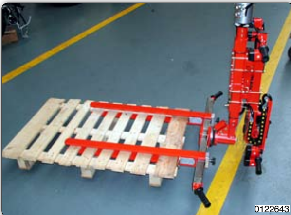
Приспособление с регулируемыми вилами и ручным поворотом груза и телескопическими элементами управления.
