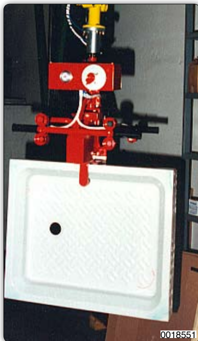
Манипулятор с пневматическим зажимом для захвата и перемещения душевых поддонов.
