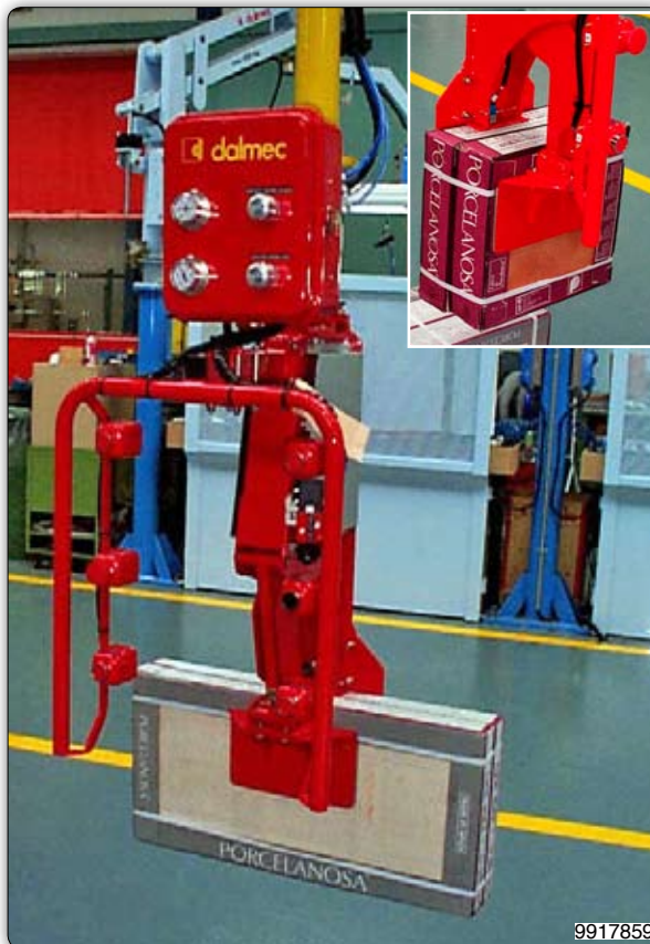
Манипулятор с приспособлением для захвата с плоскими зажимными, предназначенный для перемещения упаковок кафельной плитки.
